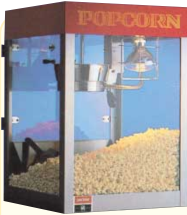
EB-002 ポップコーンマシン A サイズ:W540×D540×H780 重量:30kg 電源:100V 1325W 能力:270g/3-4分 B サイズ:W508×D368×H686 重量:20kg 電源:100V 900W 能力:270g/3-4分
